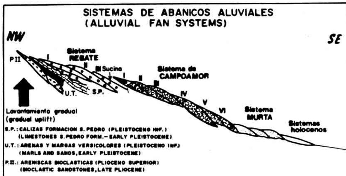
Figura 3: Dispositivo geomorfológico general de las diferentes generaciones de abanicos aluviales cuaternarios en relación con los depósitos marinos del Plioceno Superior (Según SOMOZA, 1989, GOY et al. 1989 )
