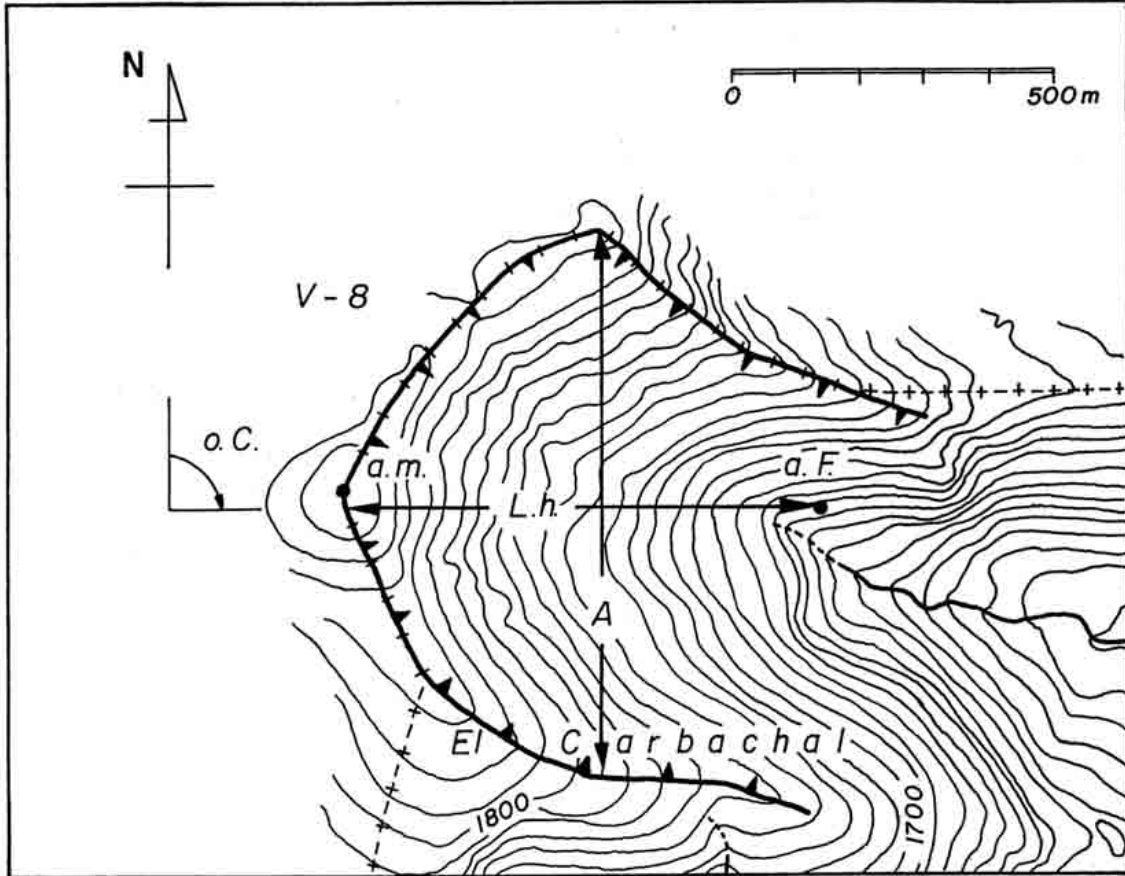
Fig. 3. Obtención de los algunos de los parámetros que caracterizan a los circos.
