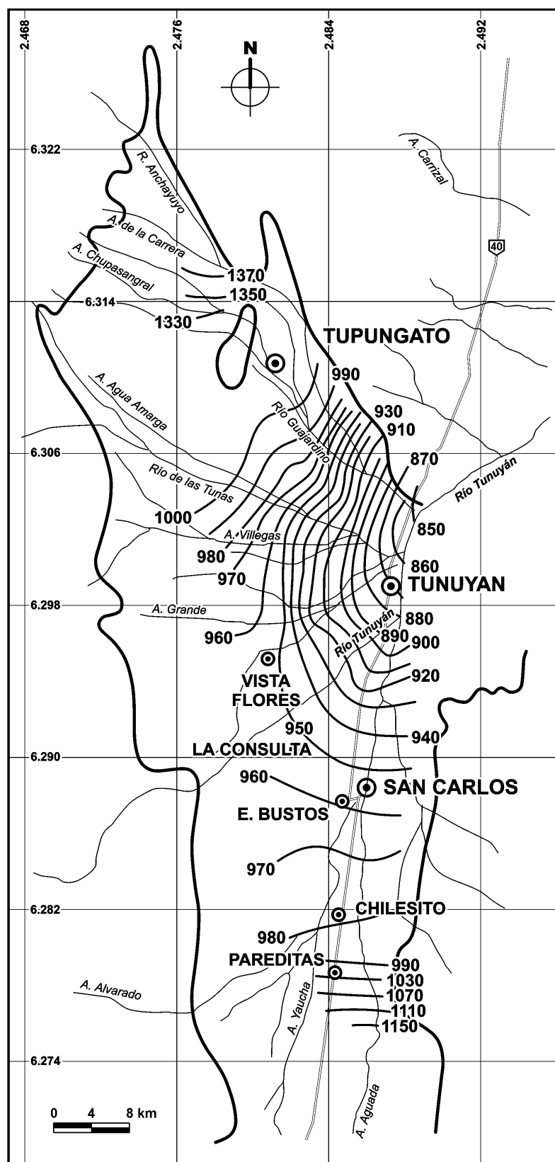
Curvas isopiezas de la zona centro.
